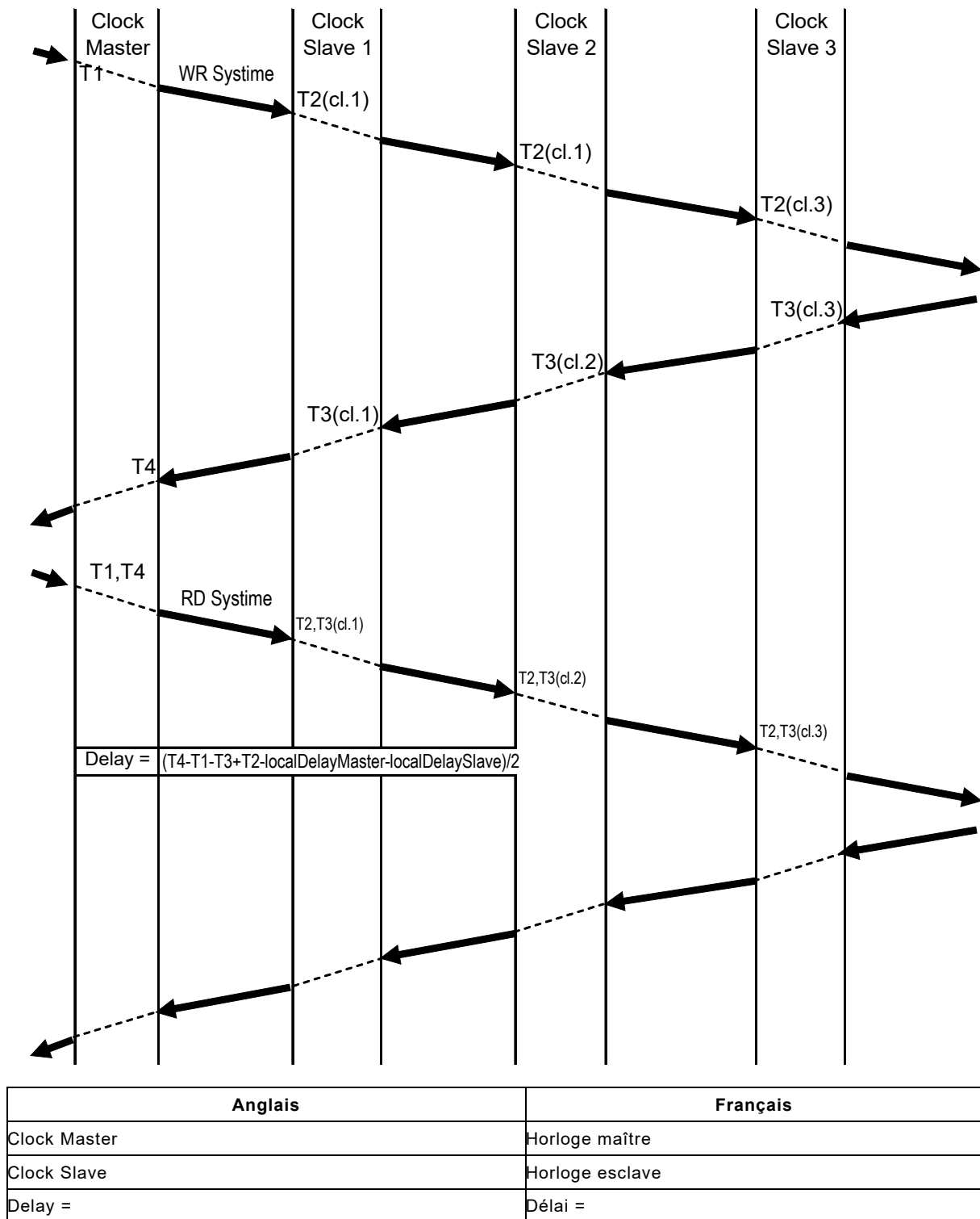
Figure 49 – Séquence de mesure du délai
