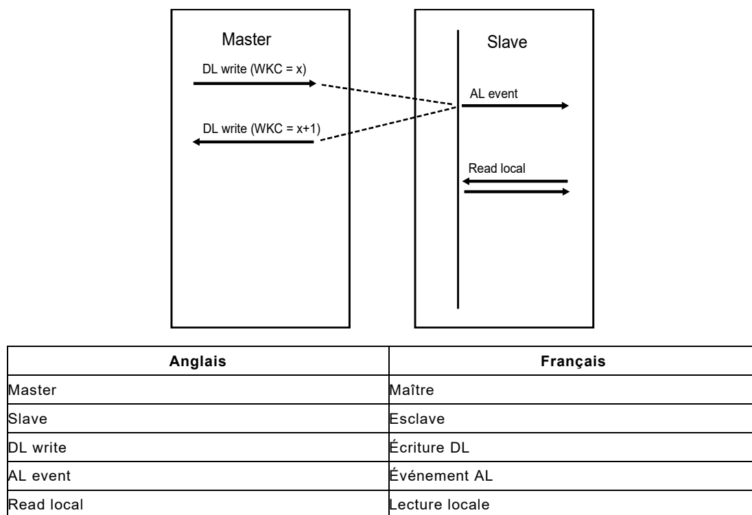
Figure 38 – Séquence d'écriture réussie dans la boîte aux lettres
